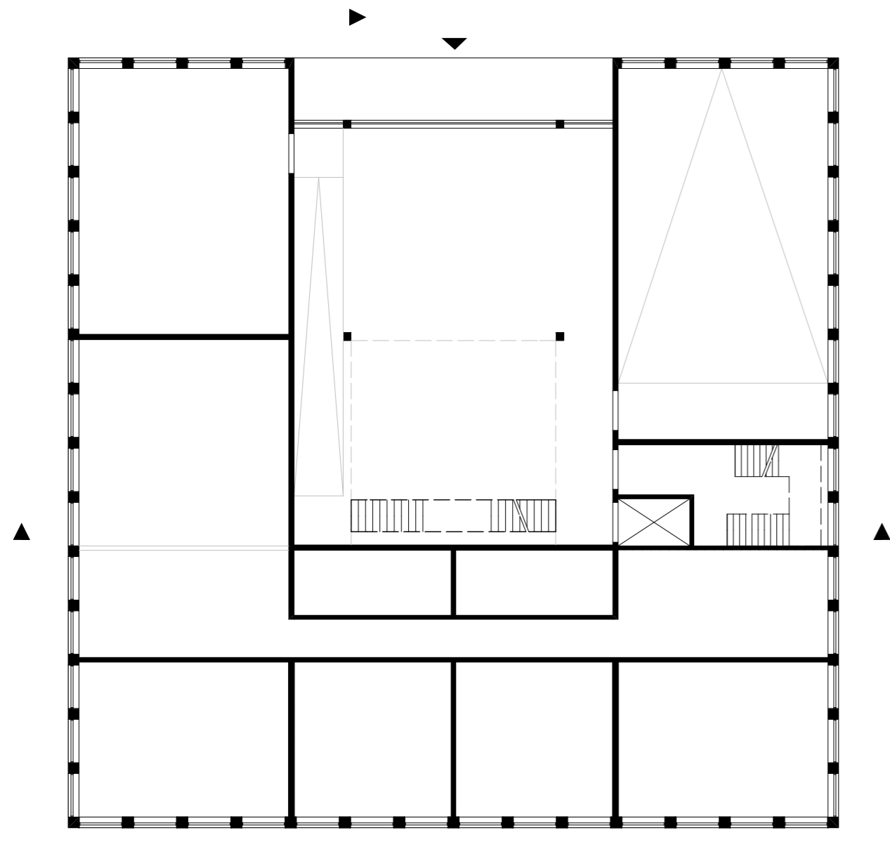
GRUNDRISS EG
