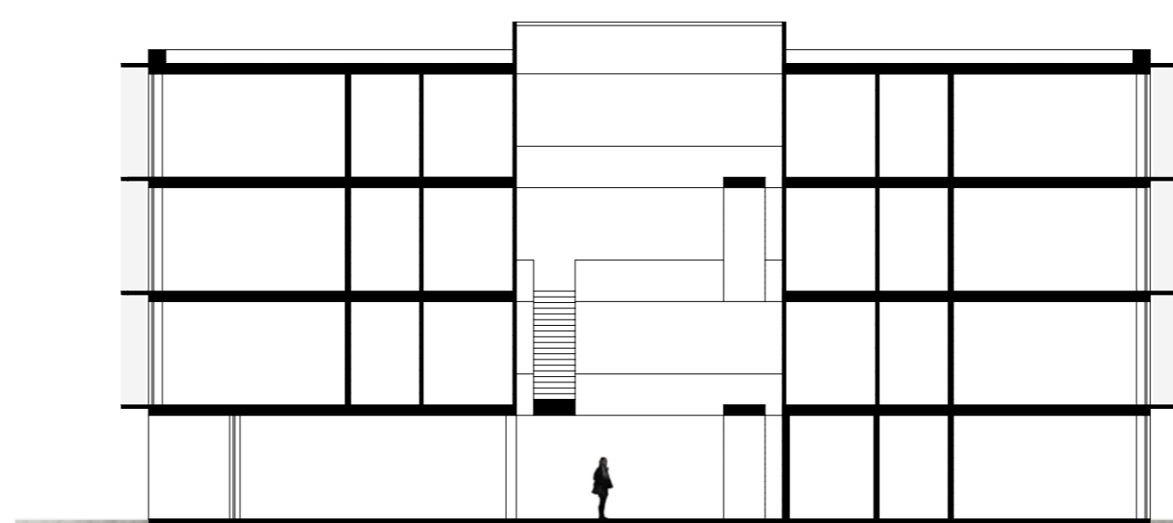
SCHNITT BB
